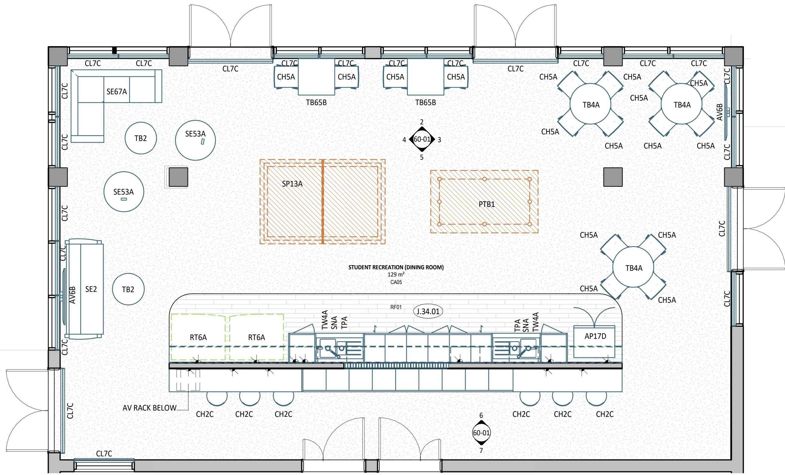
1 PLAN DETAIL 1 : 50
